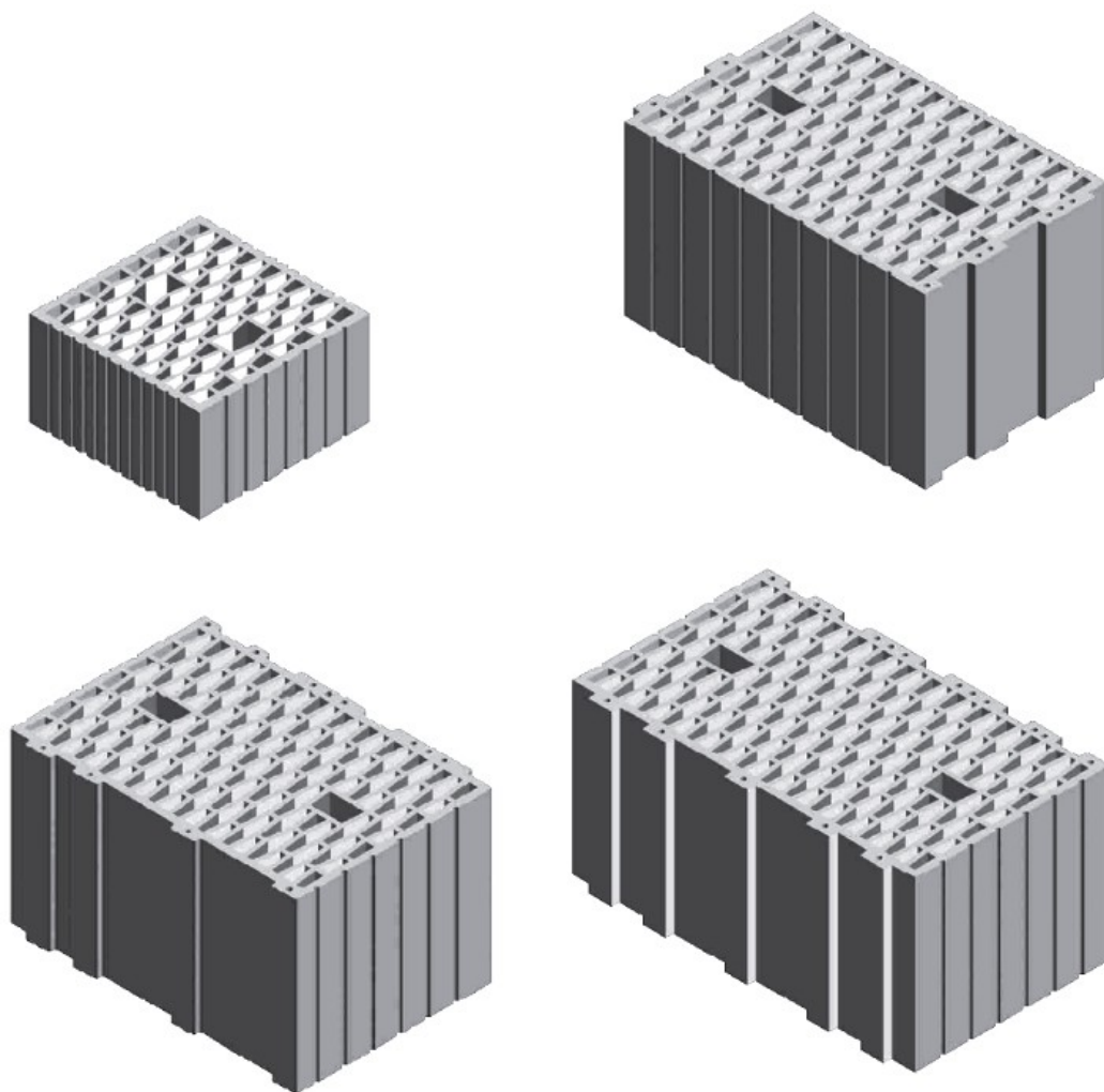
Рисунок А.4 - Камни
