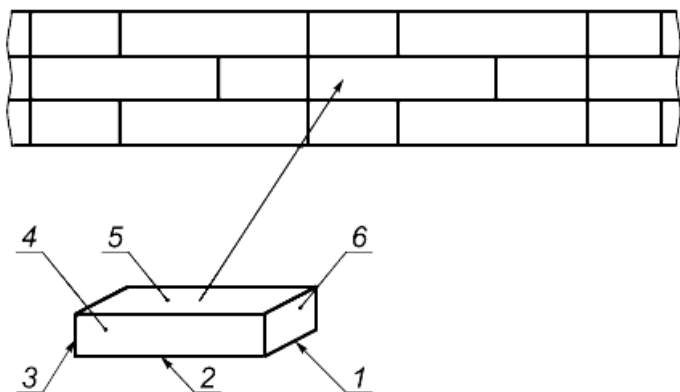
Рисунок 1 - Фрагмент кладки
